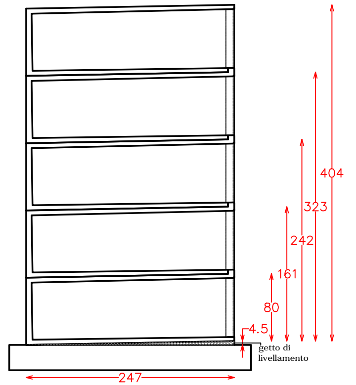
SEZIONE TRASVERSALE (fino a 5 file sovrapposte)
