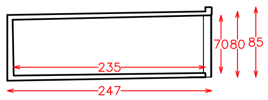
SEZIONE TRASVERSALE (singolo loculo)
