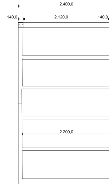
SEZIONE B-B
